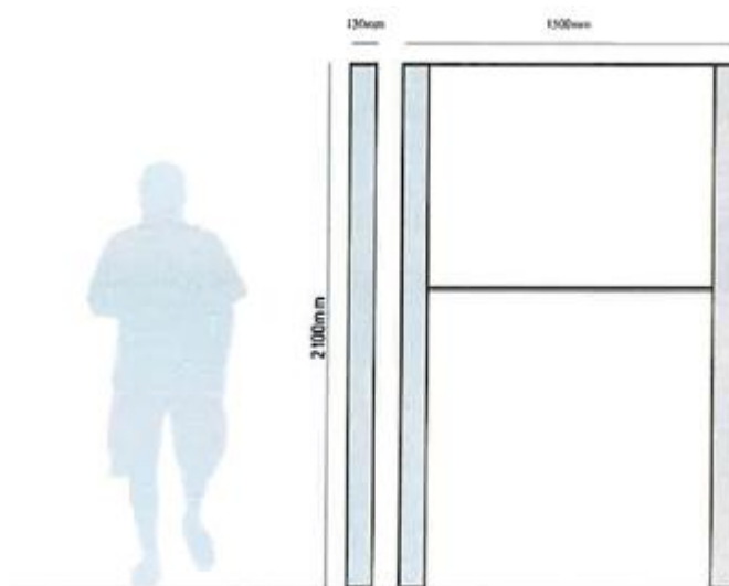
Fig. 2 - Painele informativo em estrutura em plástico reciclado
